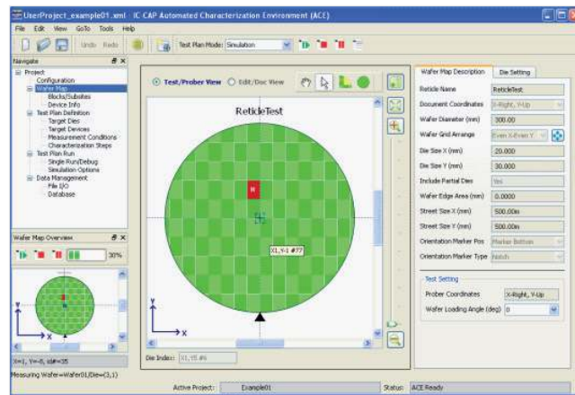
WaferPro
