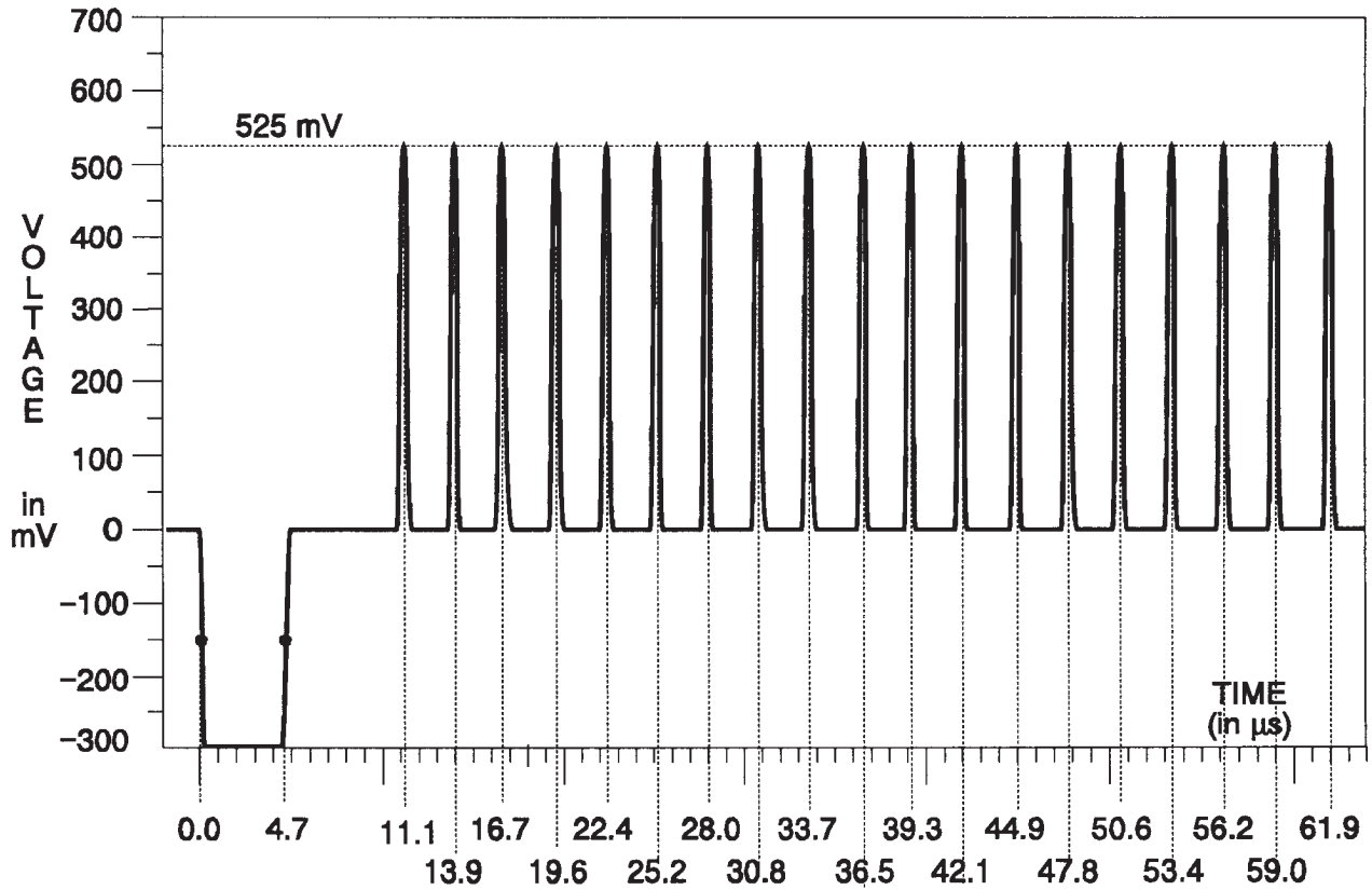
Fig. 3-127. Green Channel — Convergence (vertical).
