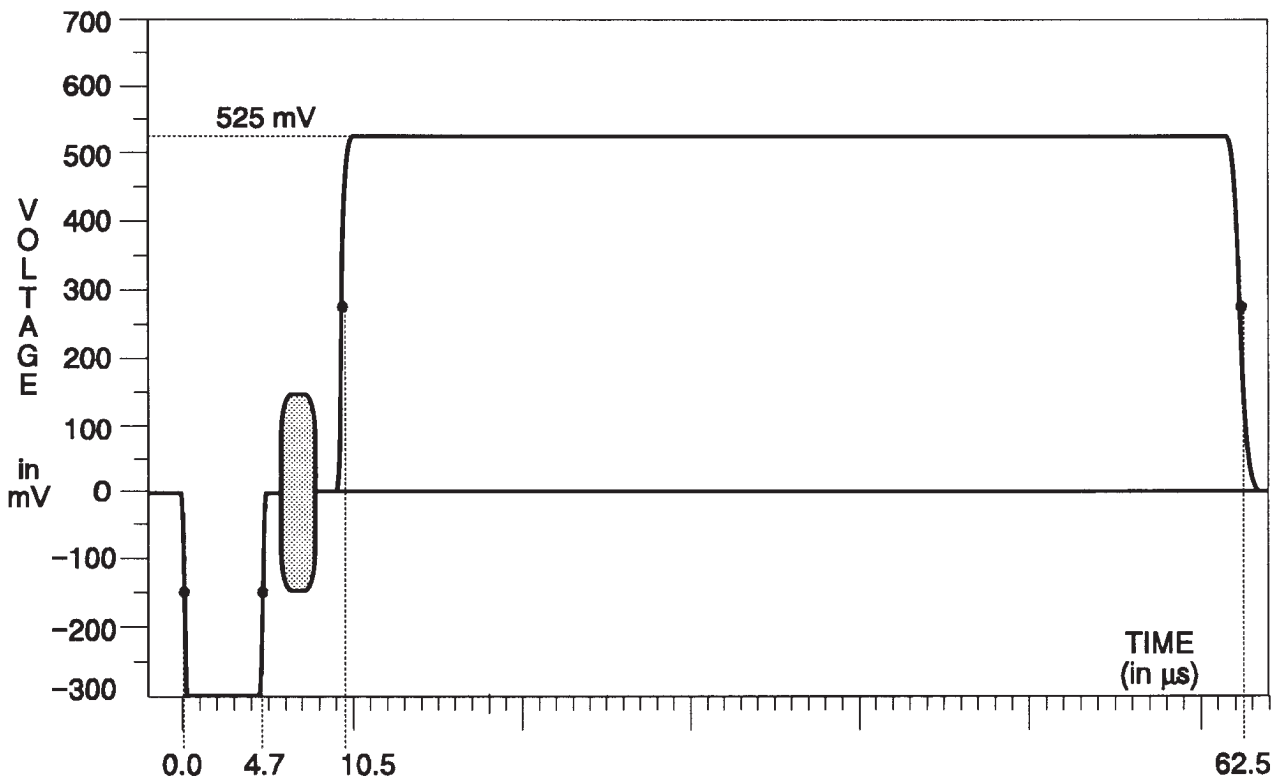
Fig. 3-14. Convergence (horizontal).
