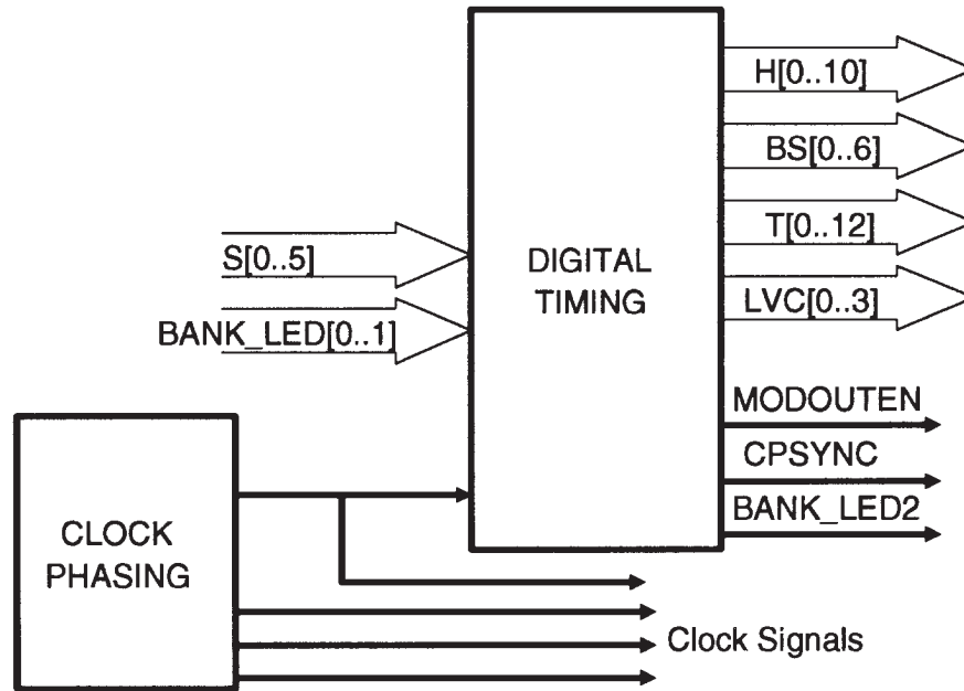
Fig. 2. Block diagram for &lt;2&gt;.
