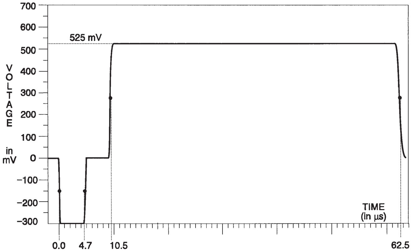
Fig. 3-69. Y Channel — Convergence (Horizontal).
