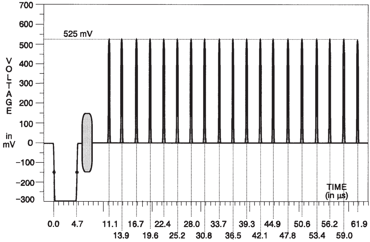
Fig. 3-15. Convergence (vertical).
