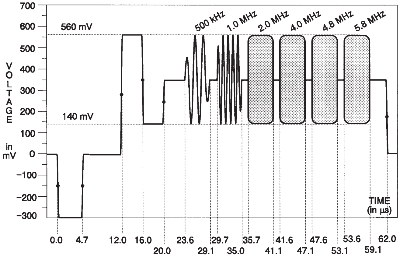
Fig. 3-62. Y Channel — Multiburst.
