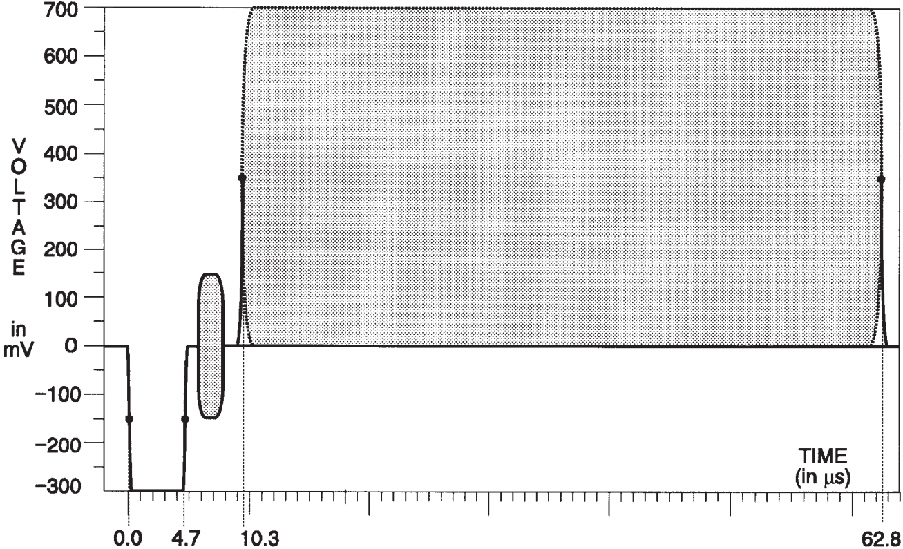
Fig. 3-12. Chroma Noise.
