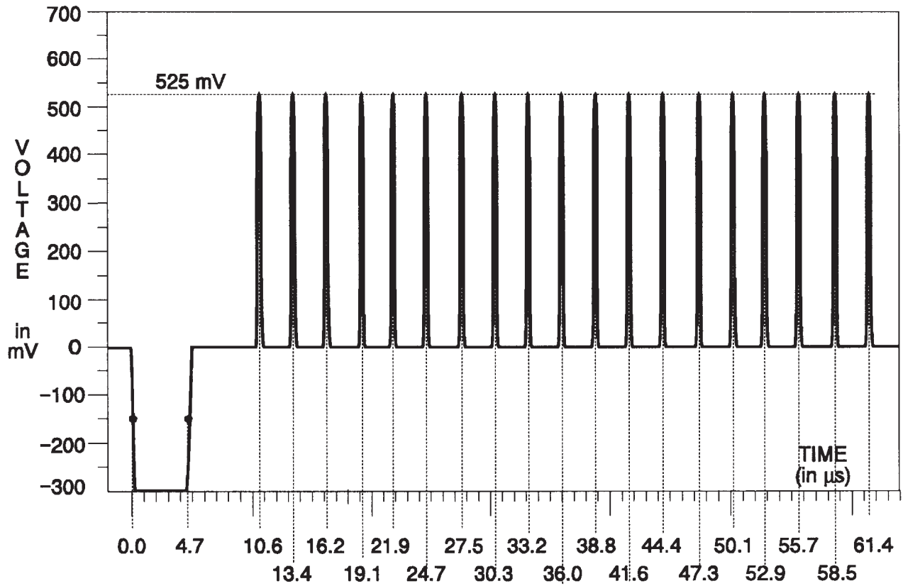
Fig. 3-173. Y Channel — Convergence (Vertical).
