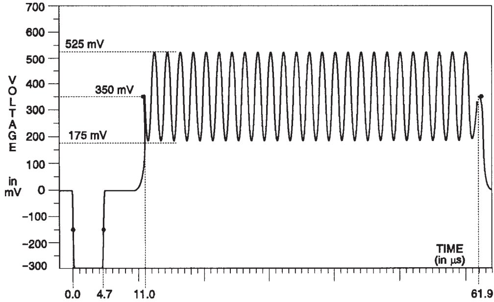
Fig. 3-98. Y Channel — Bowtie.
