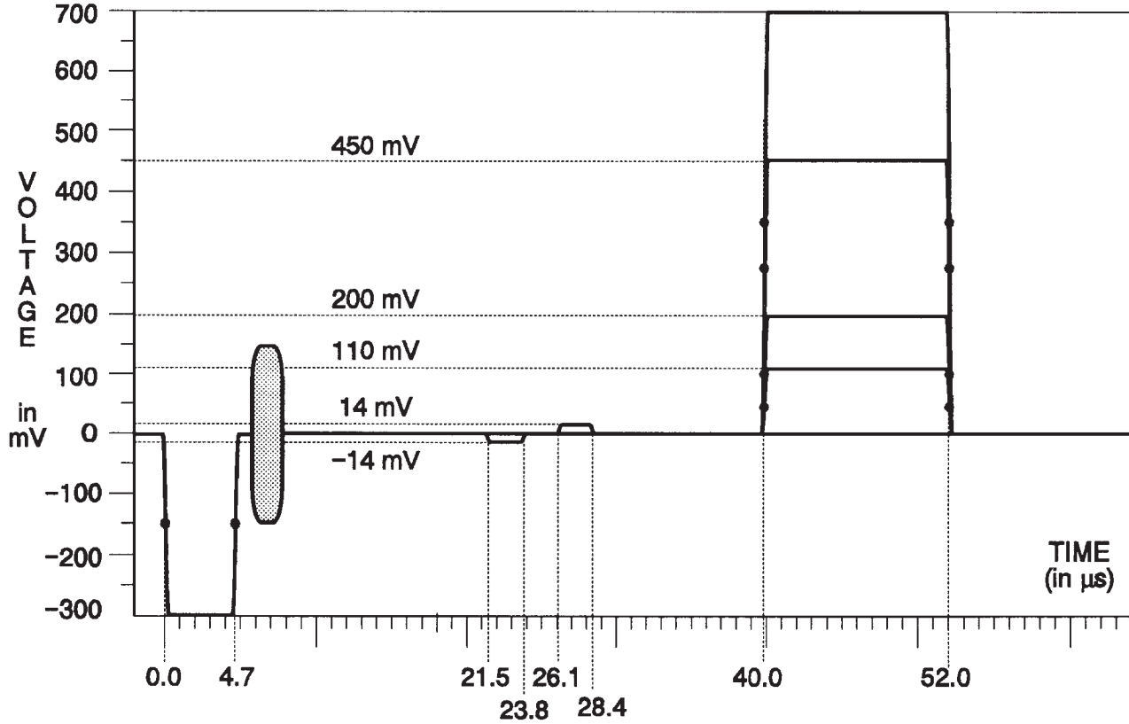
Fig. 3-22. Pluge.
