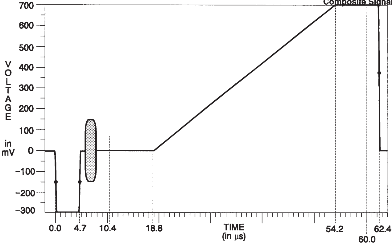
Fig. 3-16. Ramp.
