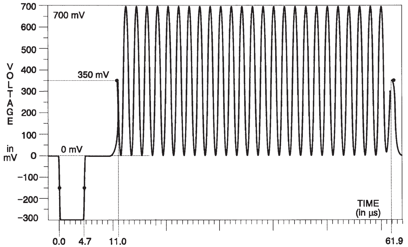
Fig. 3-239. Y Channel — 100% Bowtie.
