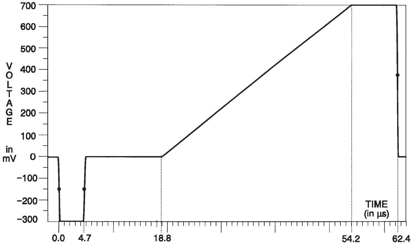
Fig. 3-58. Y Channel — Ramp.
