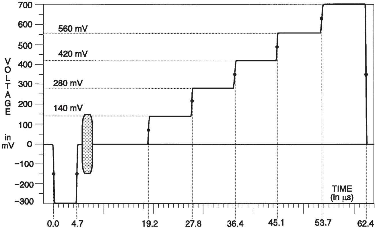
Fig. 3-13. 5-Step (Gray Scale).
