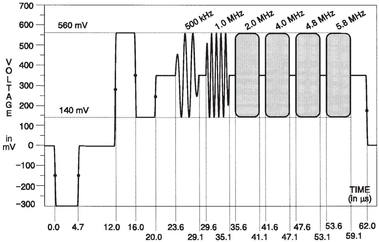
Fig. 3-215. Y Channel — Multiburst.
