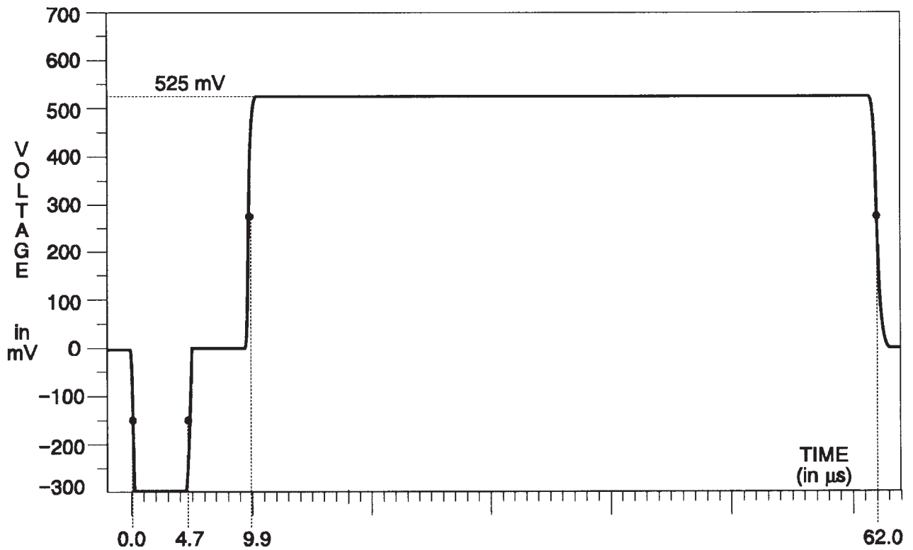
Fig. 3-174. Y Channel — Convergence (Horizontal).
