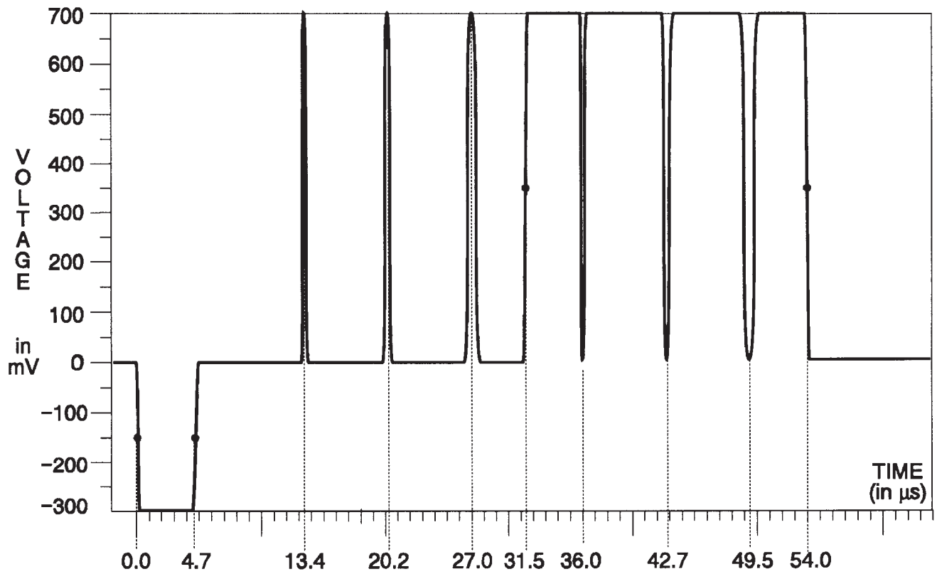
Fig. 3-195. Y Channel — T Pulses.
