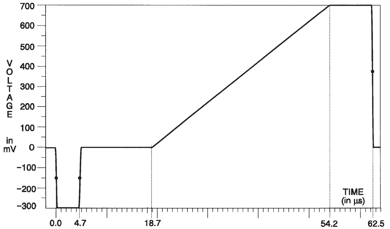
Fig. 3-217. Y Channel — Ramp.
