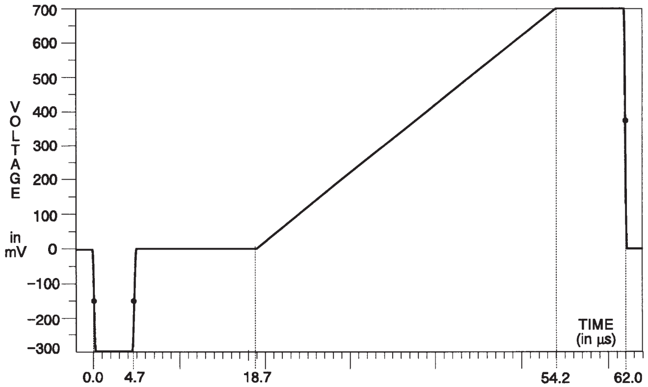
Fig. 3-167. Y Channel — Ramp.
