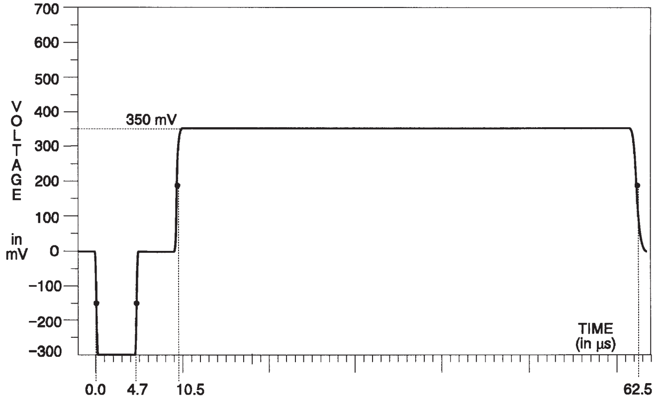
Fig. 3-52. Y Channel — Chroma Noise.
