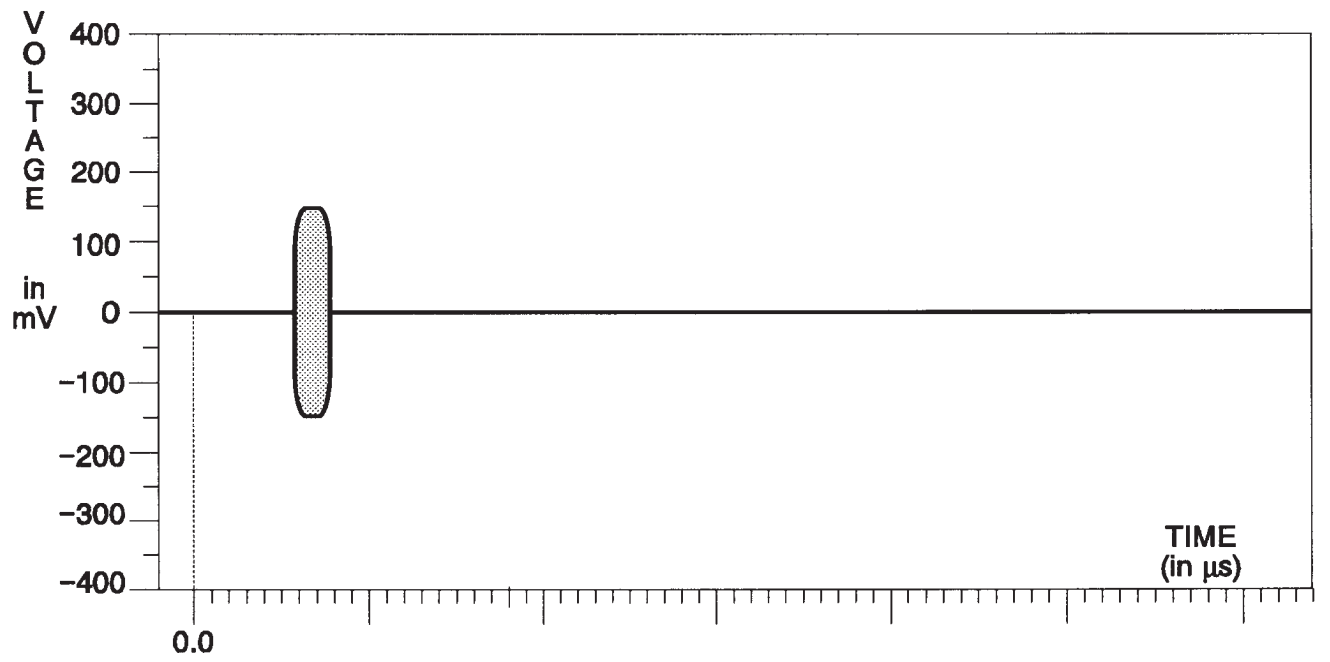
Fig. 3-218. C Channel — Ramp.
