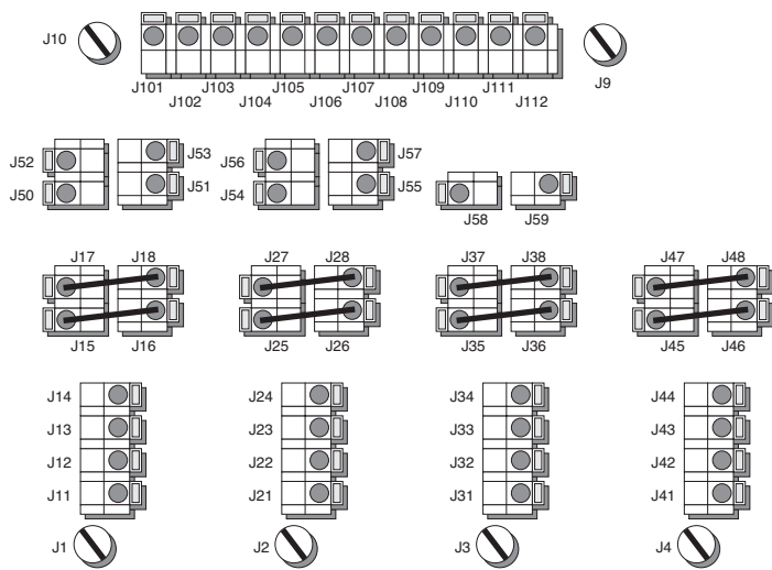
Verbindungselemente und Masseschrauben auf der Leiterplatte.
