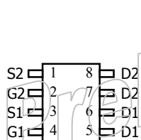
SOIC-8
